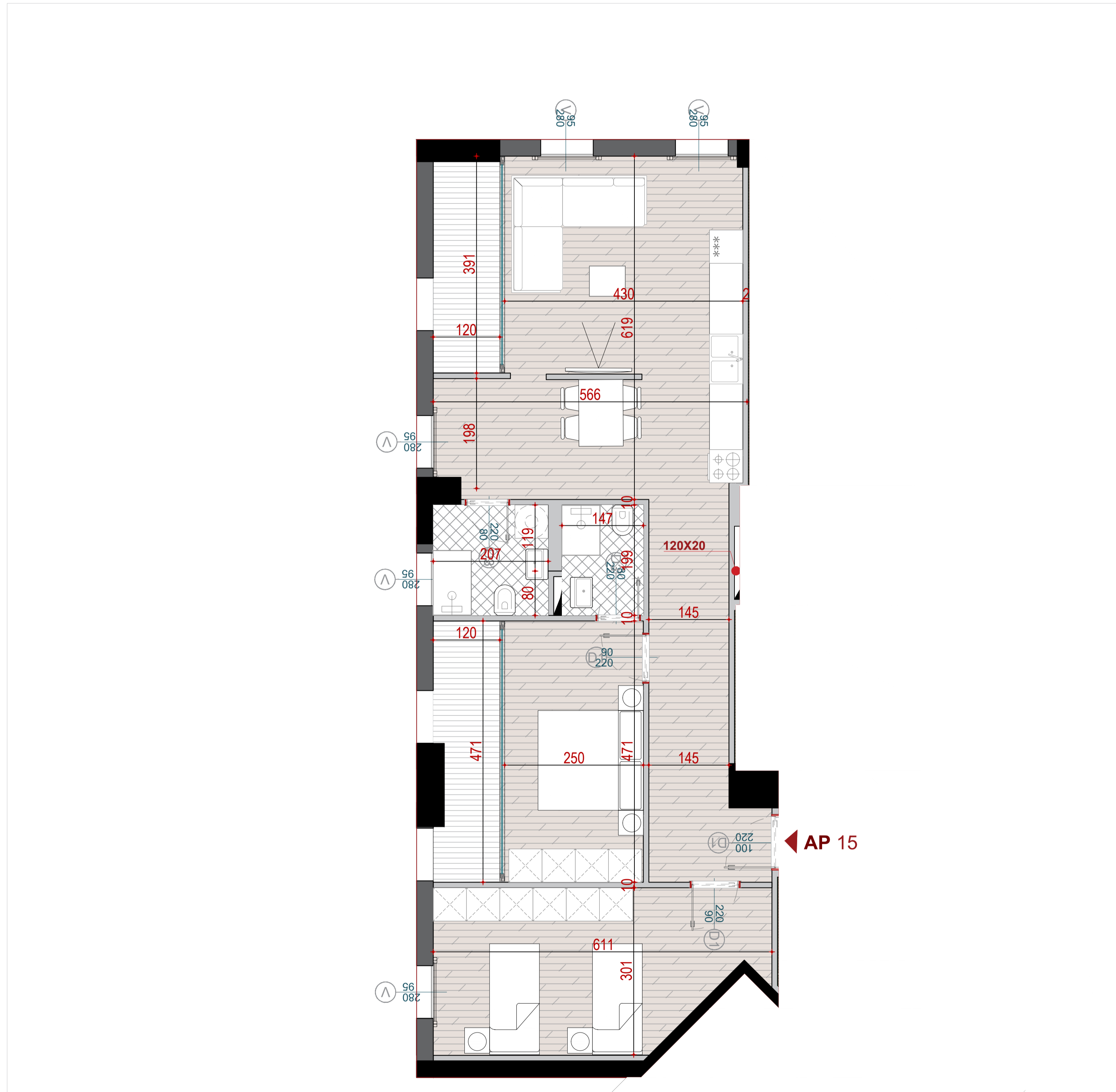
PLANIMETRIA E APARTAMENTIT NR. 15
