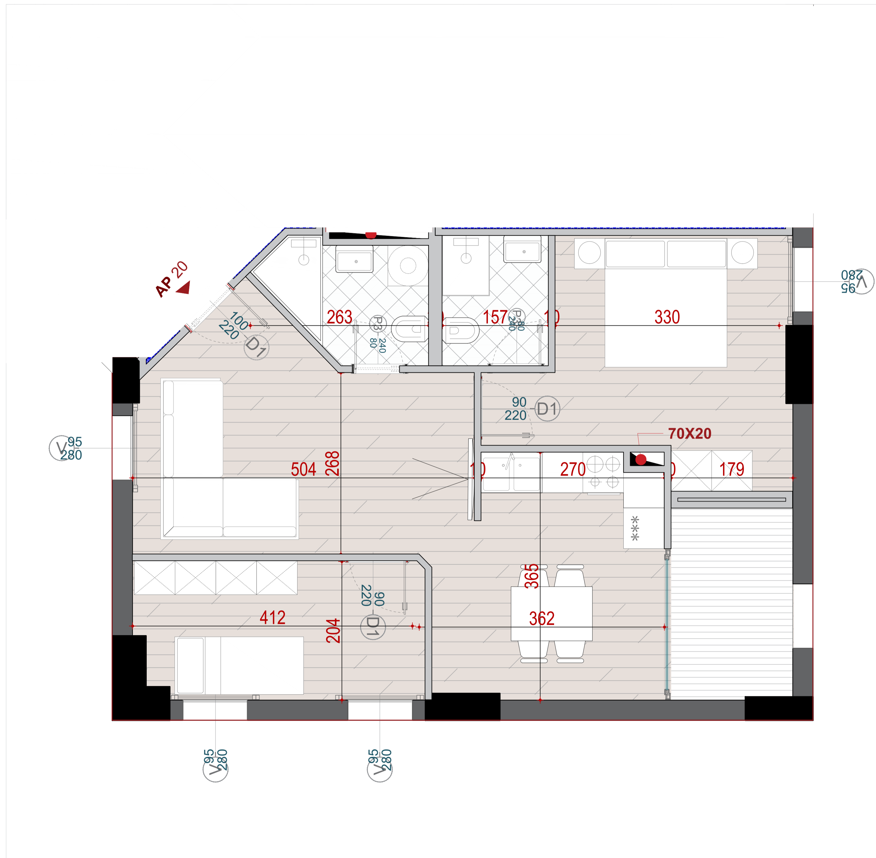
PLANIMETRIA E APARTAMENTIT NR. 20
