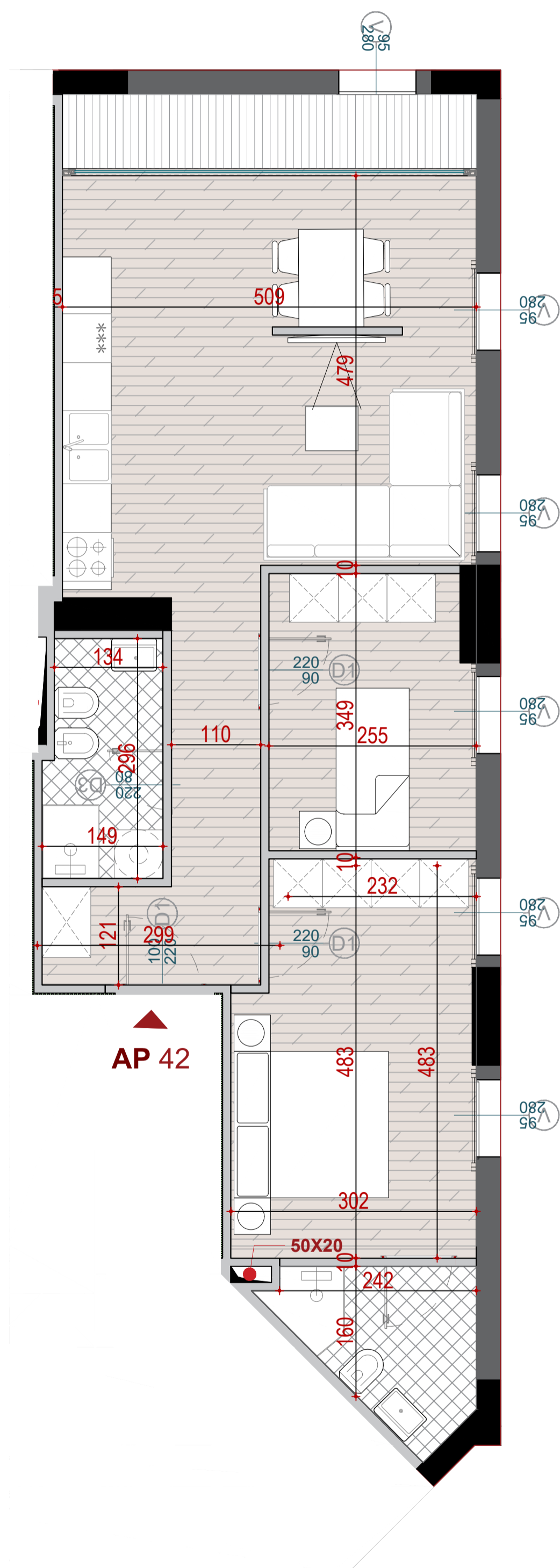
PLANIMETRIA E APARTAMENTIT NR. 42
