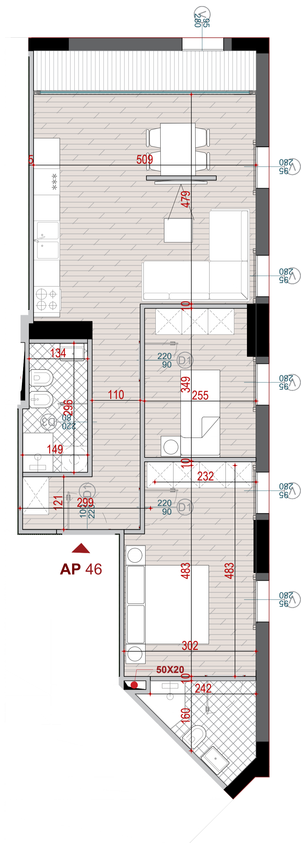
PLANIMETRIA E APARTAMENTIT NR. 46
